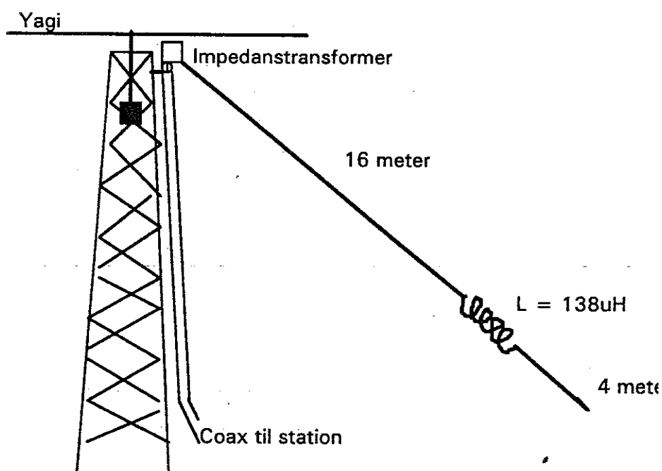
Fig.1: Forkortet sloper til 160 meter
