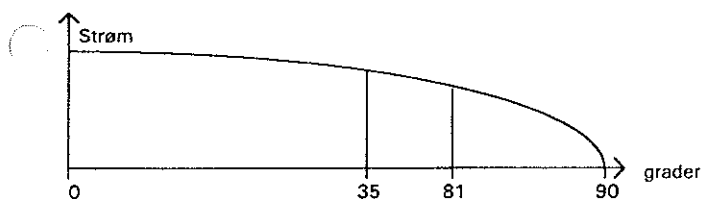
Fig. 3: Strømfordeling i antennen
