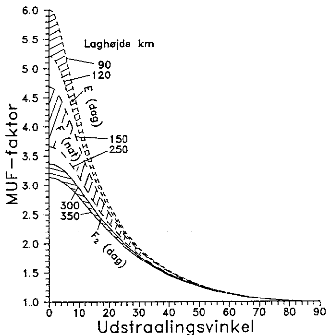
Fig. 3. MUF-faktor som funktion af udstrålingsvinkel for de forskellige ionosfærelag. For hvert lag er vist en kurve for den minimale og maksimale højde, laget kan antage. MUF = Maximum Usable Frequency.
