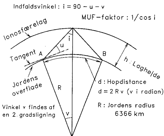
Fig. 1. Hopdistance ved radiobølgers udbredelse via ionosfæren. Ionosfærelagets højde er stærkt forstøret.
