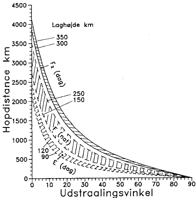
Fig. 2. Hopdistance som funktion af udstrålingsvinkel for de forskellige ionosfærelag. For hvert lag er vist en kurve for den minimale og maksimale højde,
