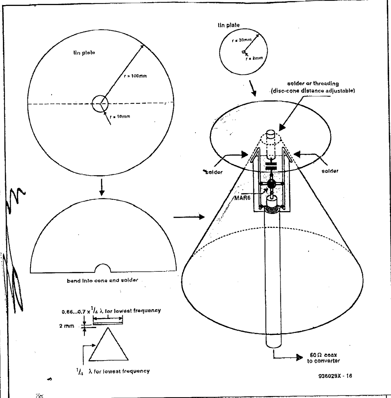
Figur 15. Dimensioner och konstruktionsdetaljer för skivkon-antennen.
